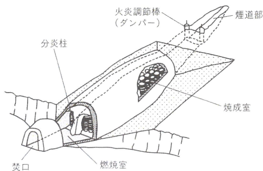
窯室模式図 (山茶碗専焼窯)
