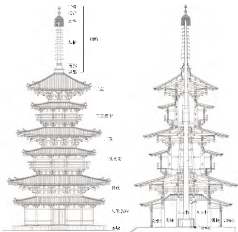
東塔の各部名称
