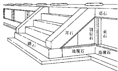
階段の模式図
