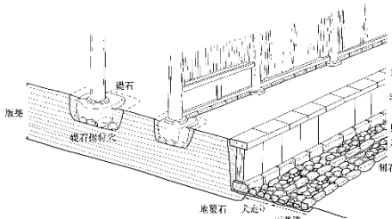
基壇および基壇周辺の模式図
