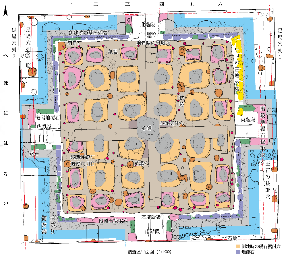
調査区平面図 (1:100)
